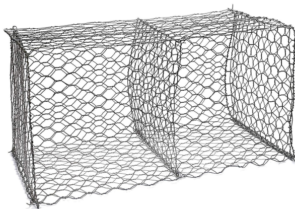
图 5-2 铅丝石笼
