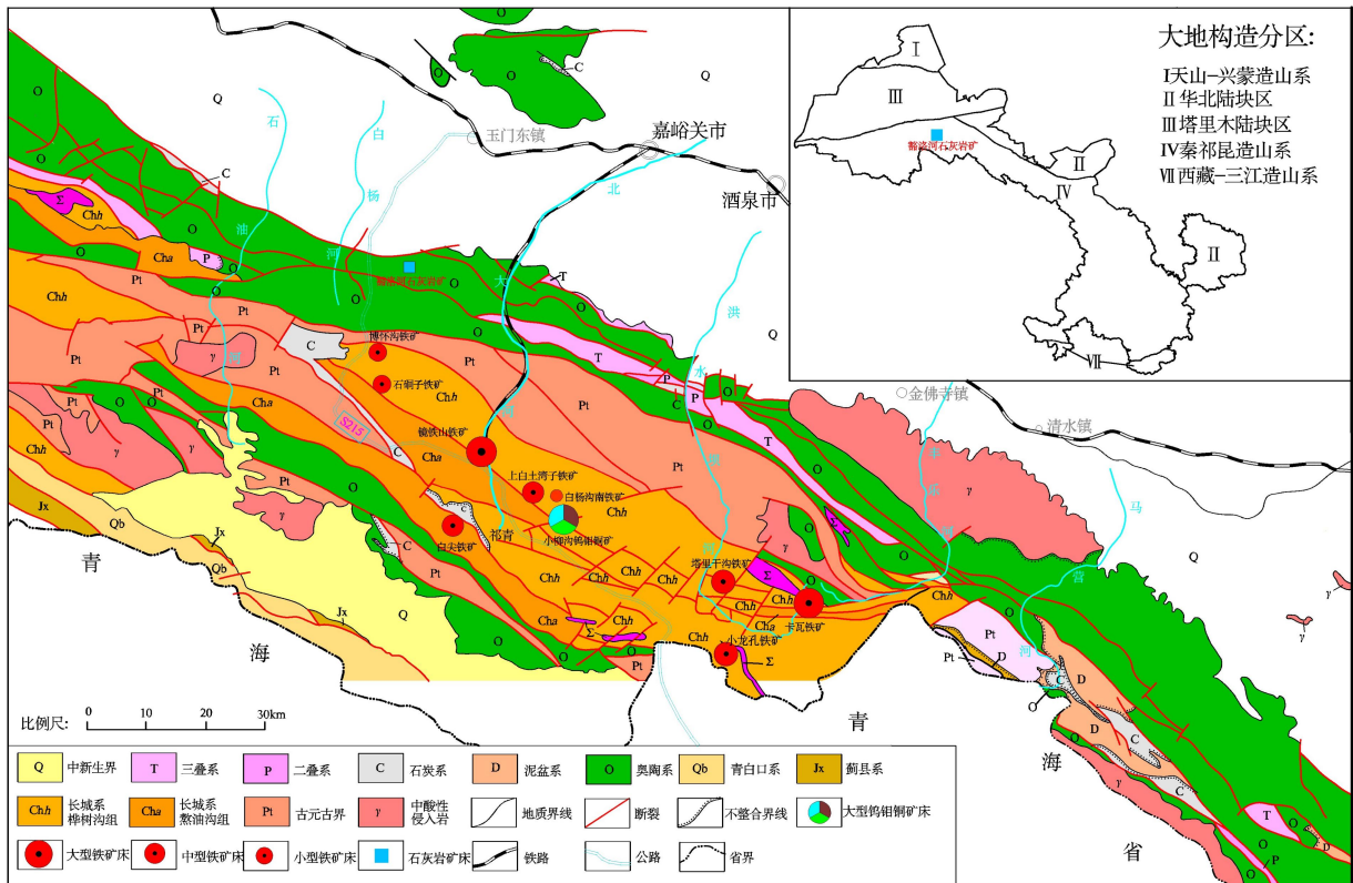
图 3-1 矿区区域地质简图
