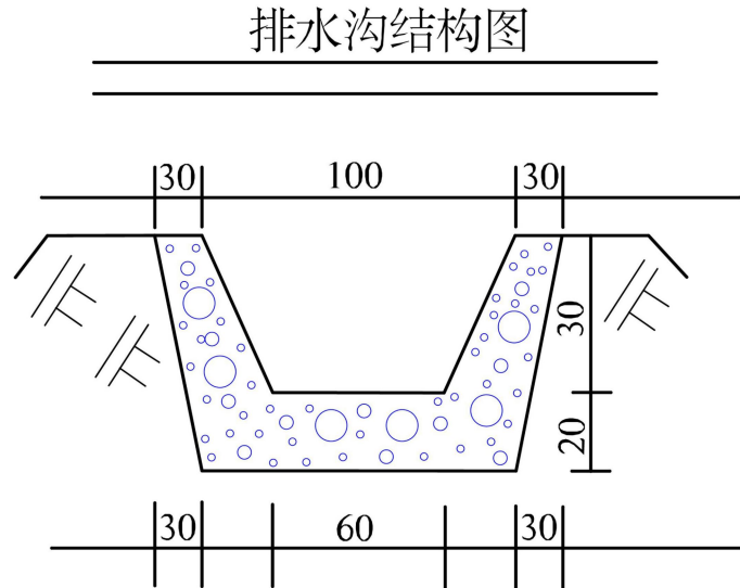
图 5-3 排水沟结构图
