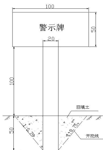
图 5-1 警示牌设计图
